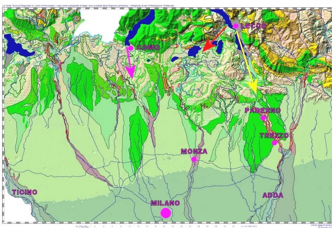
Fig. 2. Carta geologica della Lombardia in cui è possibile vedere il tracciato attuale del fiume Adda (freccia gialla), quello antico che scaricava dal varco di Malgrate (freccia rossa) e l'antichissimo sbocco del fiume Paleoadda, che scaricava dal ramo di Como, più di un milione di anni fa (freccia viola)
