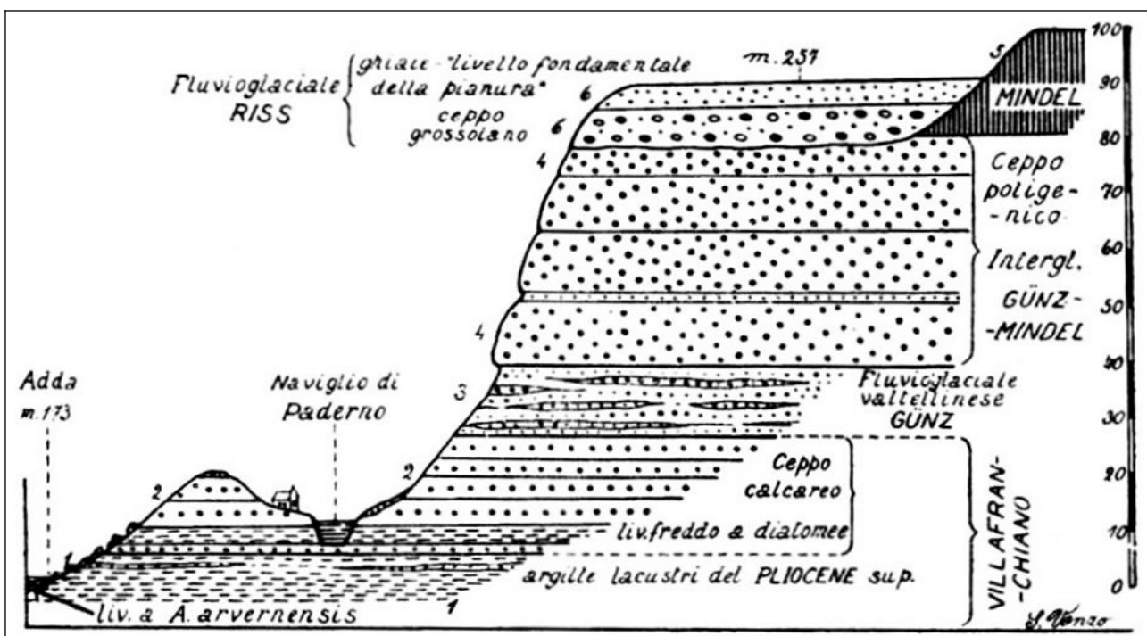
Fig. 6. Stratigrafia geologica della sponda destra dell'Adda all'altezza di Paderno, inserita nell'articolo, disegnata e descritta dal Prof. Venzo. L'immagine è tratta dalla rivista Atti della Società Italiana di Scienze Naturali (1950)
