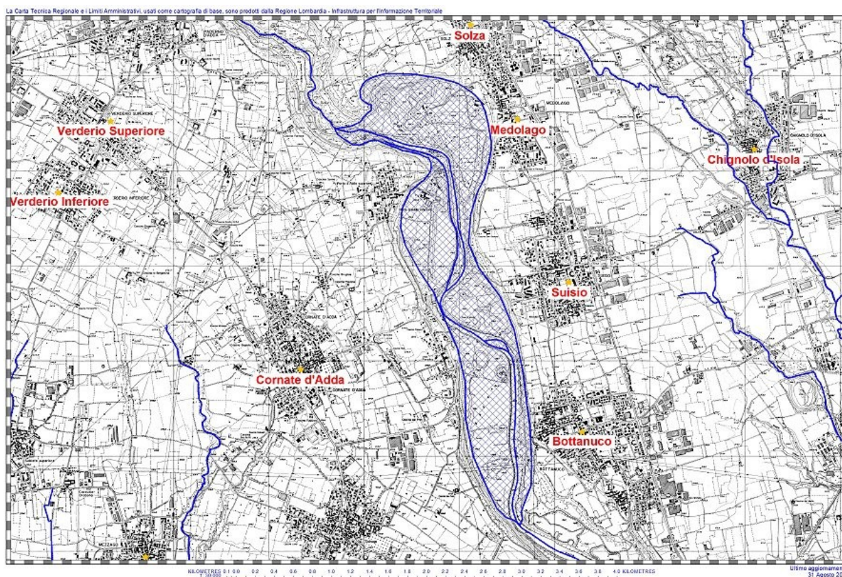
Fig. 8. Le altimetrie delle località poste a Nord di Trezzo indicano chiaramente che, se il livello dell'acqua dell'Adda fosse poco più elevato di quello attuale (152 m s.l.m. a Trezzo), ciò sarebbe sufficiente per creare un invaso tra i paesi di Bottanuco, Suisio e Medolago per quanto riguarda la sponda bergamasca e tra Colnago, Cornate e Porto d'Adda per quella milanese
