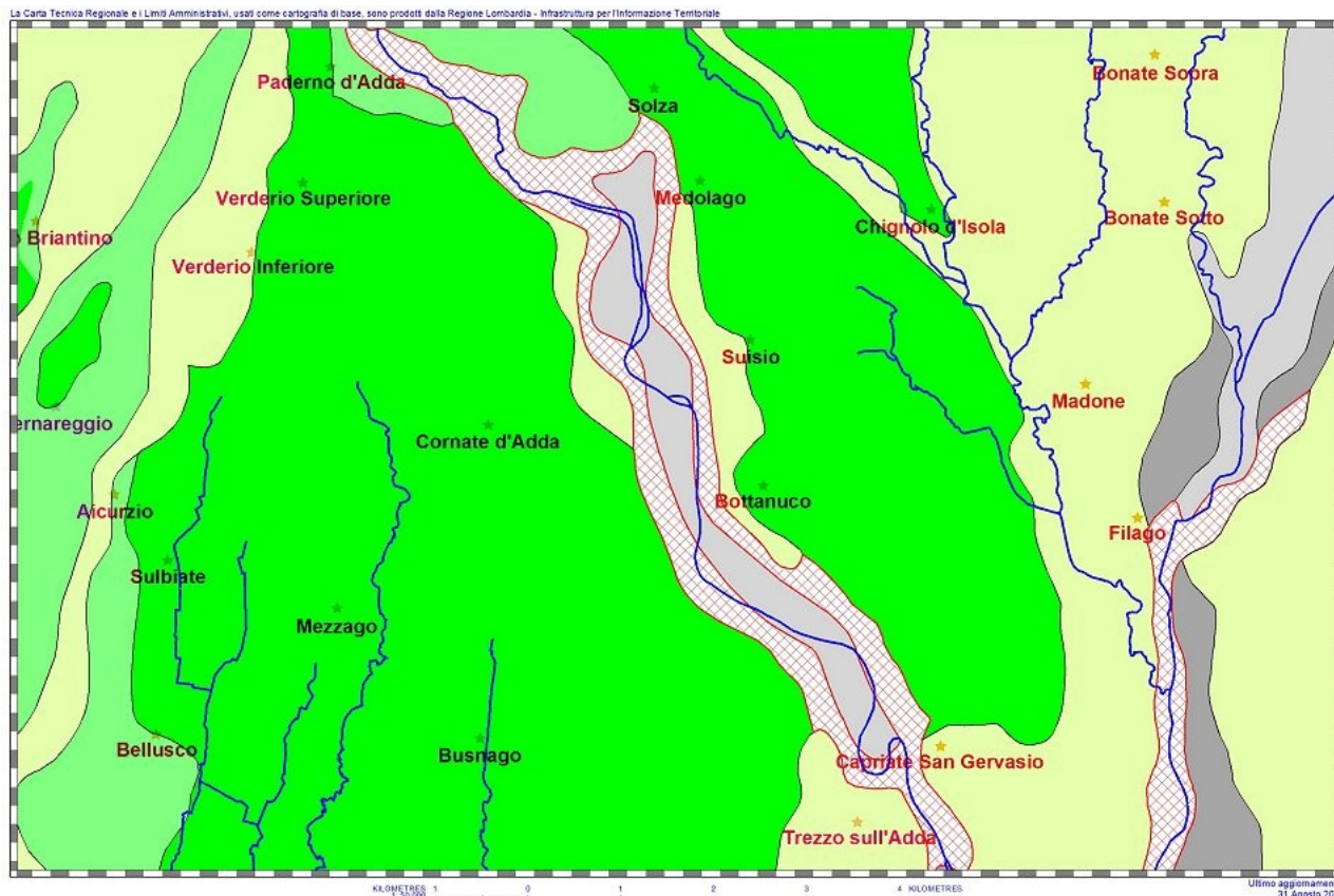
Fig. 7. Stralcio della carta geologica in cui risulta evidente la continuità nella formazione del ceppo tra Paderno e Trezzo sull'Adda, indicata dall'area con il reticolo a rombi. L'alveo del fiume ha inciso profondamente da Nord a Sud il terrazzo mindelliano (verde vivo), mettendo in luce la stratigrafia del canyon dell'Adda, nella quale il ceppo ha una potenza di parecchie decine di metri. A destra, si nota la presenza dello stesso sostrato di ceppo anche lungo il letto del Brembo, in questo caso direttamente sotto il Livello Fondamentale della Pianura (LFdP, in verde pastello), nel territorio bergamasco
