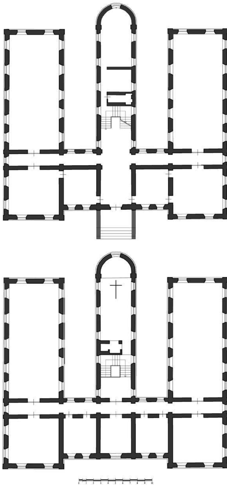
7. Pianta del piano terra rialzato e del primo piano con l'eliminazione delle superfetazioni moderne (arch. Antonio Giovannoni).
