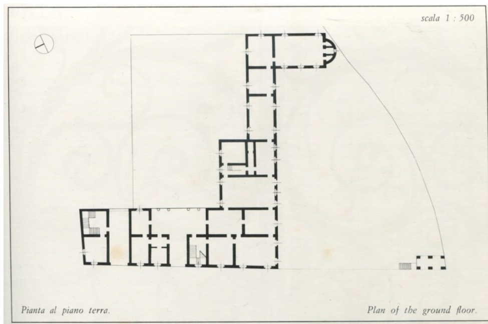
Pianta del piano terreno (da C. Perogalli e P. Favole, Ville dei navigli lombardi)
