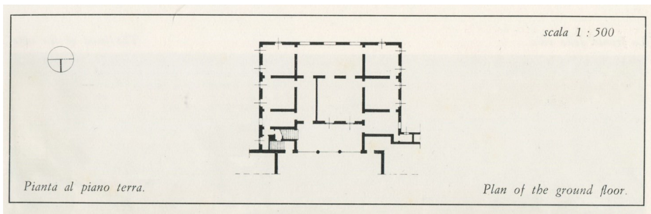
Pianta del piano terreno (da C. Peregalli e P. Favole, Ville dei navigli lombardi)
