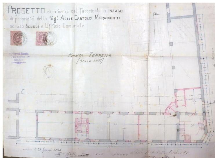
Mappa piano terra
